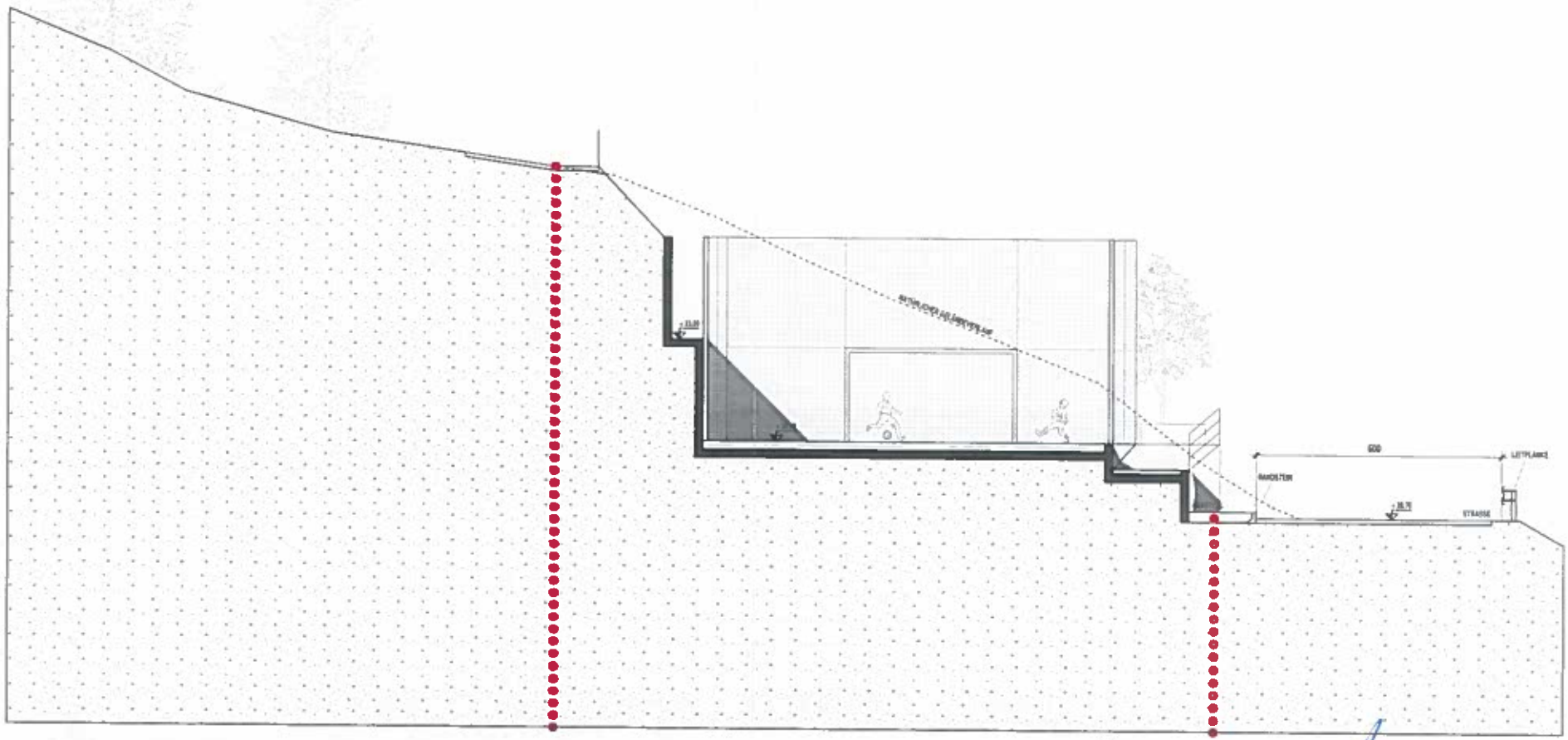
SCHNITT A-A
