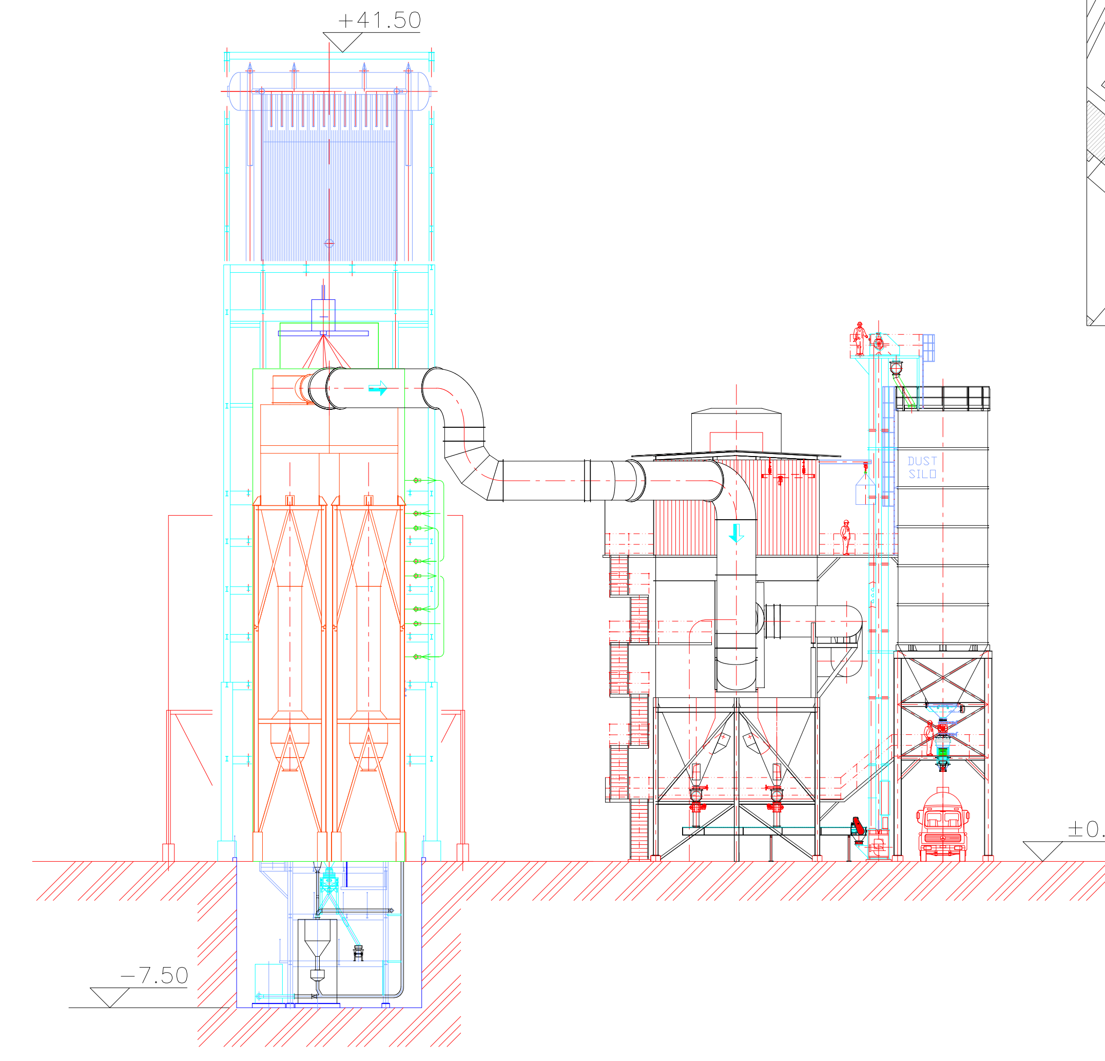
VISTA C-C
