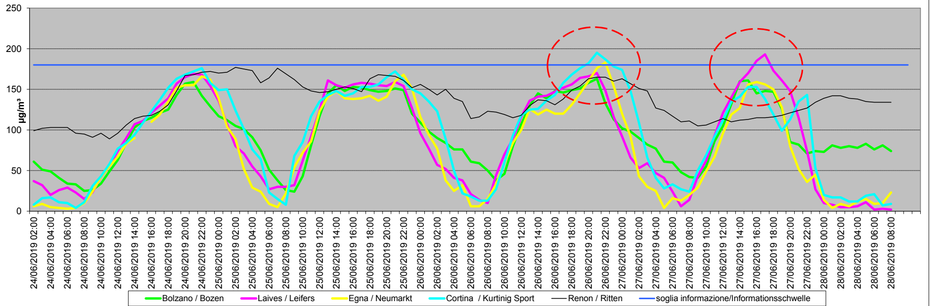
Medie orarie dell'ozono 24-27 giugno 2019 Ozon-Stundenmittelwerte 24.-27. Juni 2019
