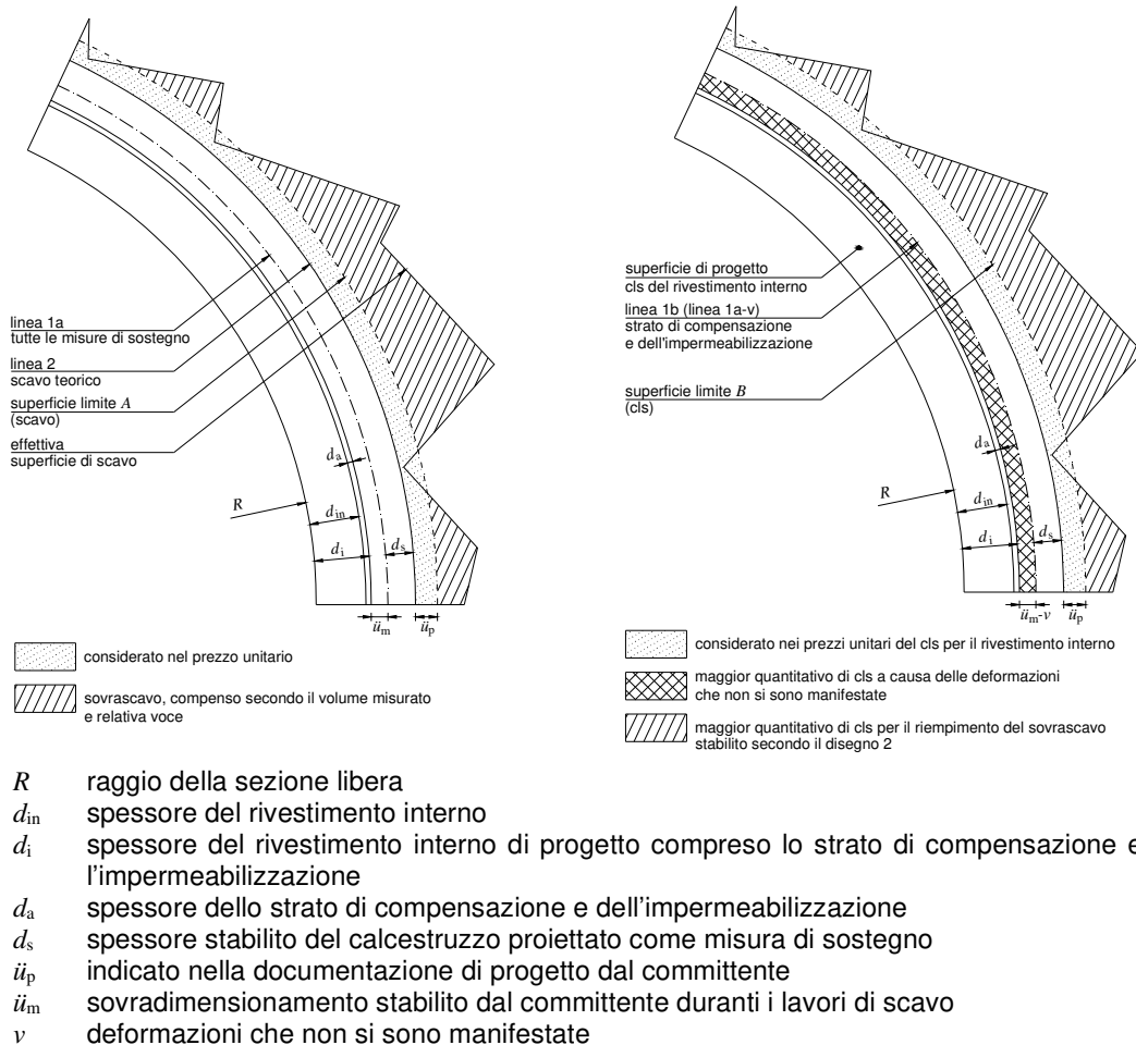
Figura 2: Linee di contabilizzazione; scavo e opere di sostegno – Rappresentazione prima delle deformazioni
