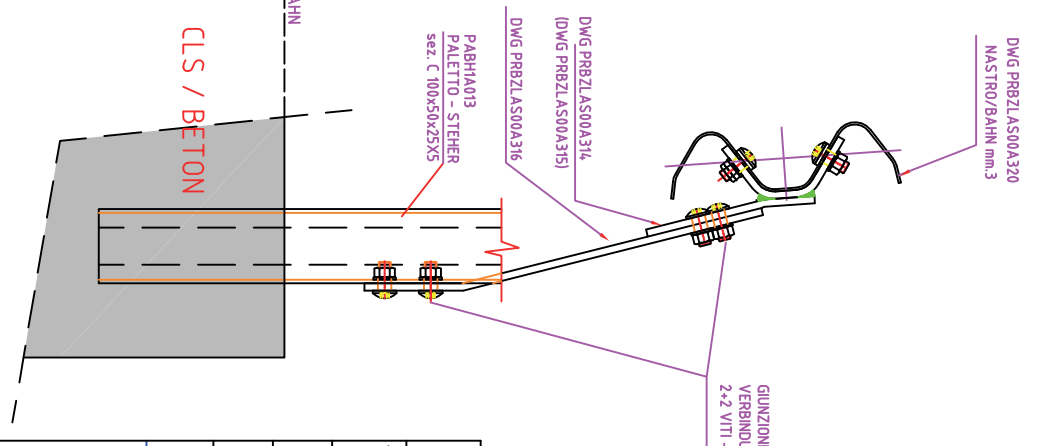
SEZIONE B-B SCHNITT SCALA / M 1:10
