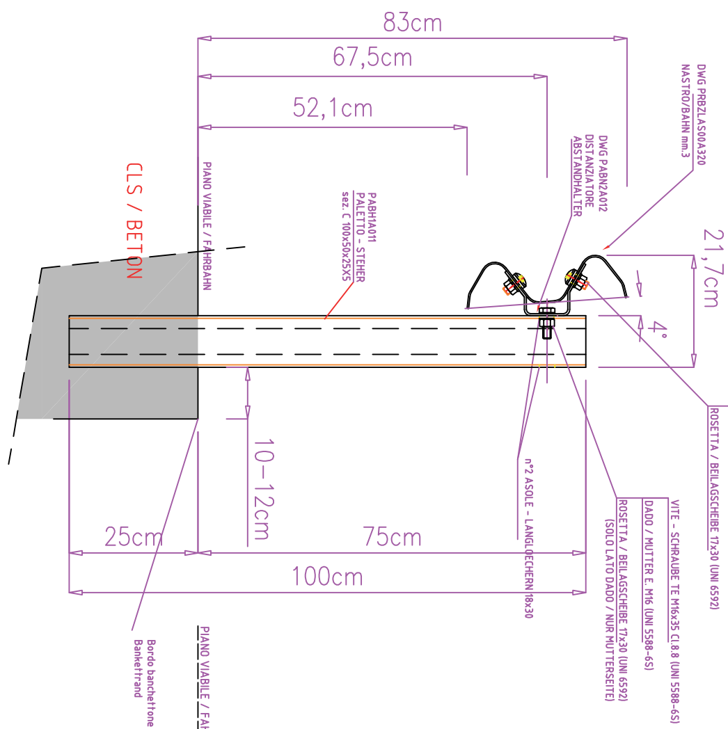
SEZIONE A-A SCHNITT SCALA / M 1:10
